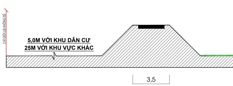
MẶT CẮT 4 - 4
