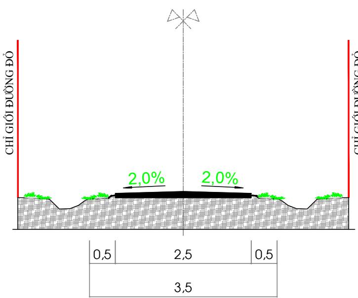
MẶT CẮT 3 - 3
