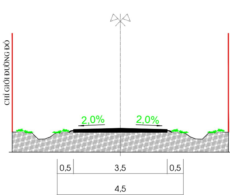
MẶT CẮT 2 - 2
