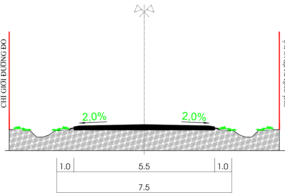
MẶT CẮT 1 - 1
